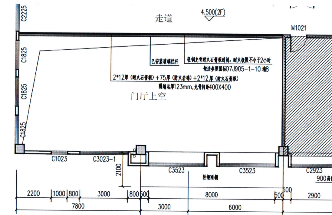
二层玻璃走道与一层大厅隔断(后期需拆除)
