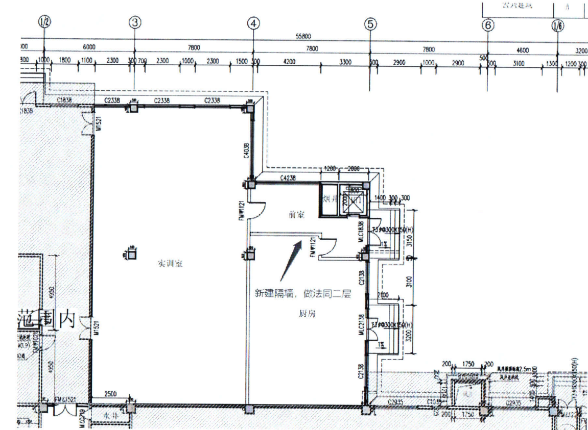
一层烹饪实训室与传菜电梯之间隔断
